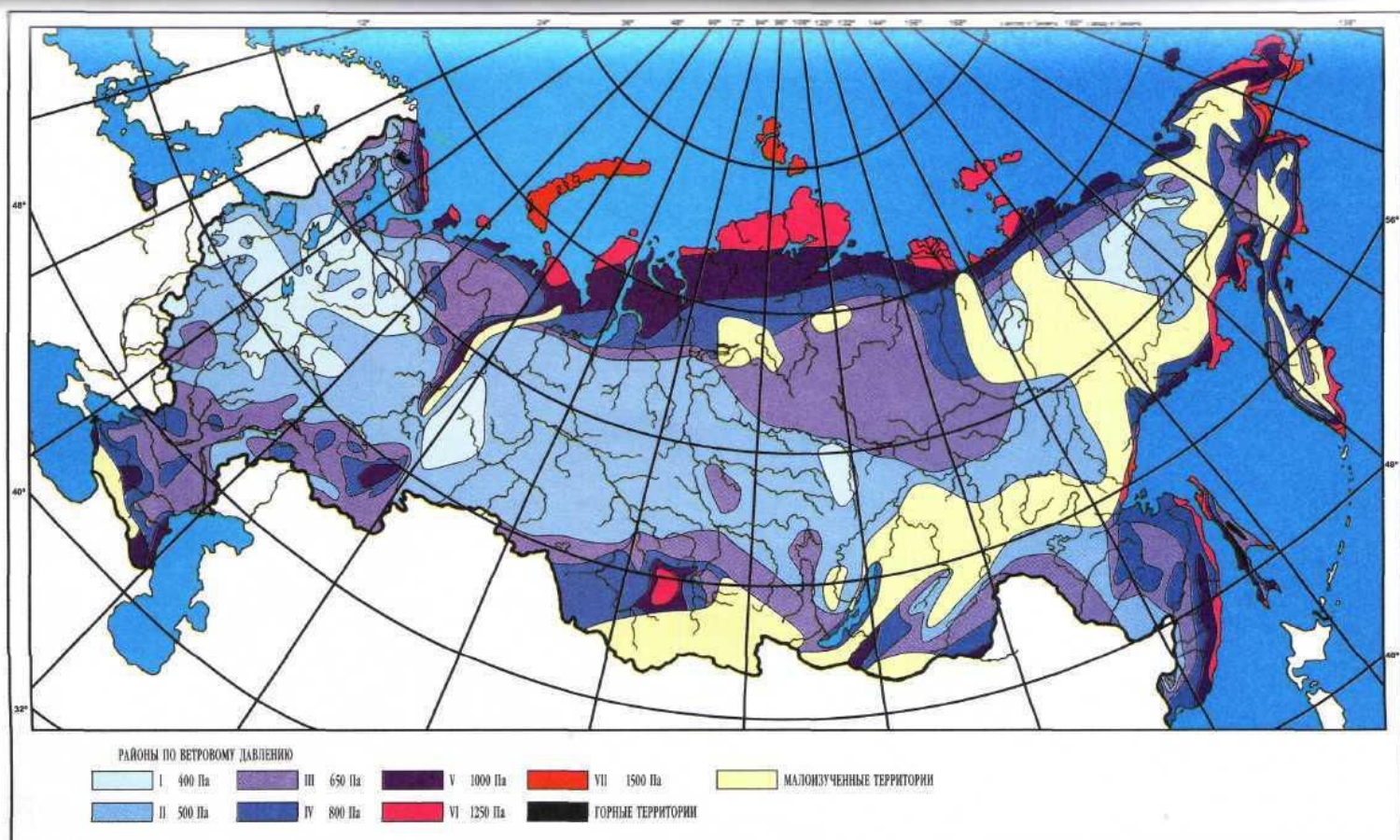
Рис. 2.5.1. Карта районирования территории РФ по ветровому давлению
